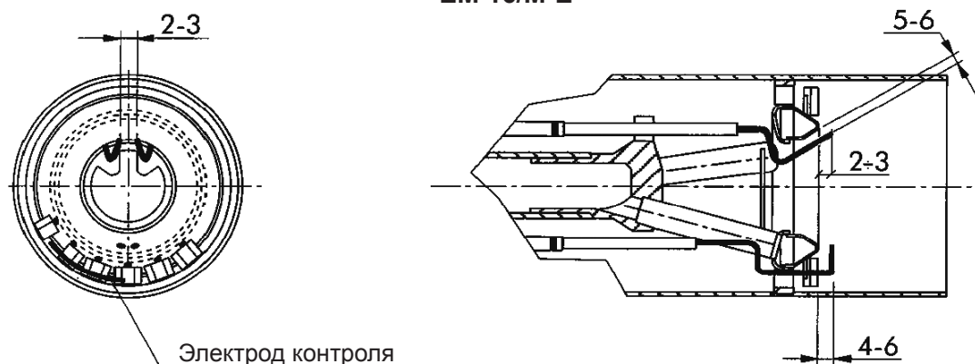
ЕМ 16/М-Е
