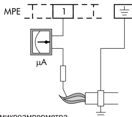
Присоединение микроамперметра
