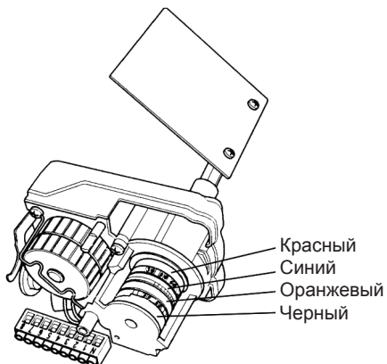
Сервопривод типа SQN 70 ...
