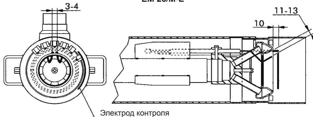
ЕМ 26/М-Е
