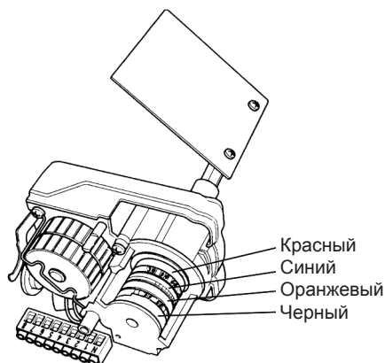
Сервопривод типа SQN 70 ...
