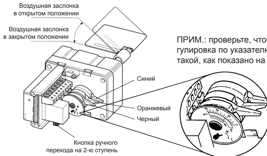
Сервопривод типа CONECTRON LKS 120
